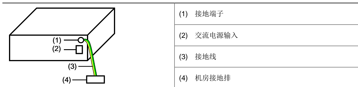
图2-13 接地安装示意图（机房有接地排）
