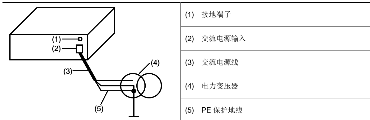
图2-15 接地安装示意图（利用交流 PE 线接地）
