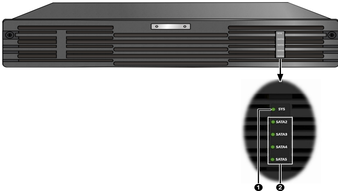
图1-4 前面板指示灯
