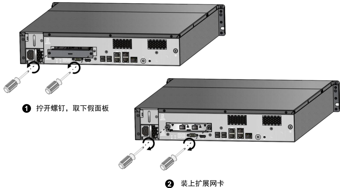
图2-10 安装扩展网卡
