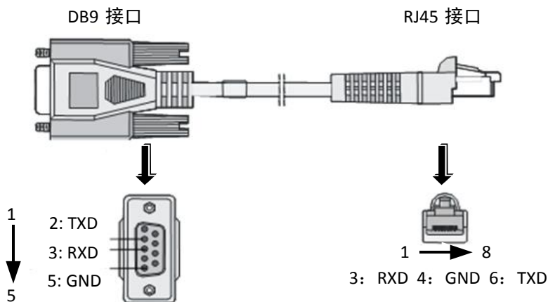
图2-11 RS232 串口线
