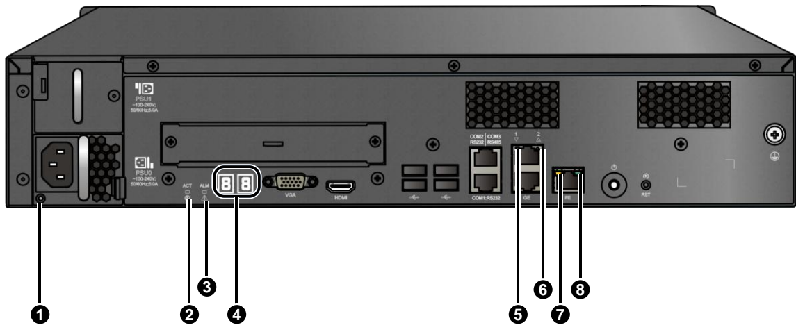
图1-5 后面板指示灯/数码管
