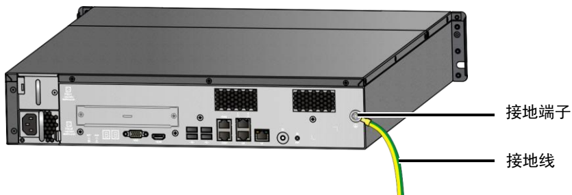
图2-12 接地线连接示意图
