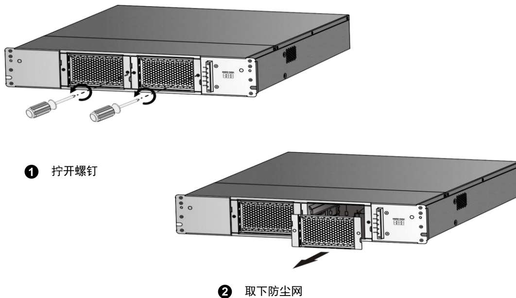
图2-6 拆卸防尘网
