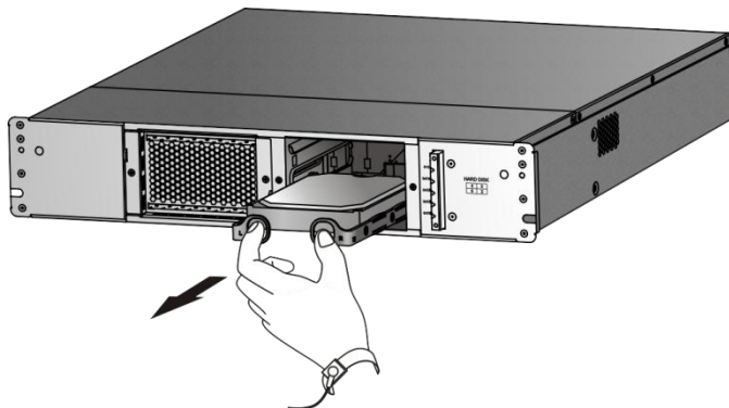
图6-1 拔出硬盘
